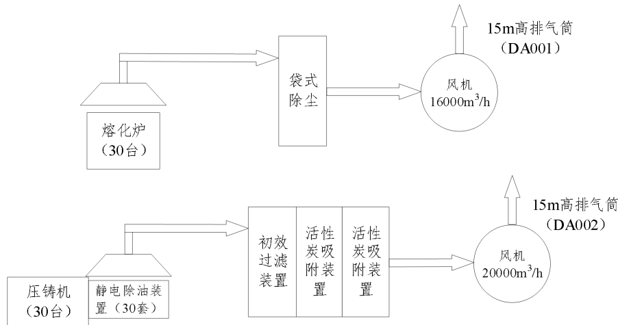
图 4-1 本项目废气处理工艺示意图
