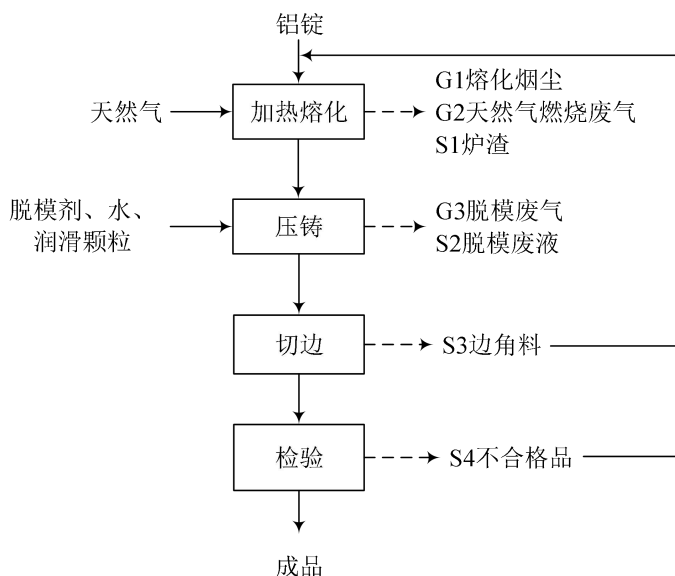
图 2-7 生产工艺流程图
