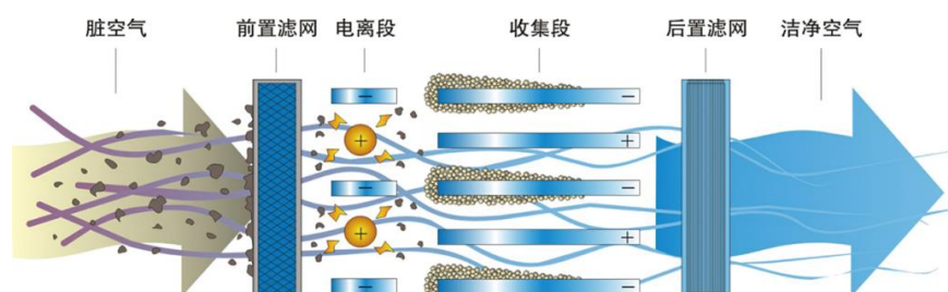
图 4-3 油雾净化工艺流程示意图
