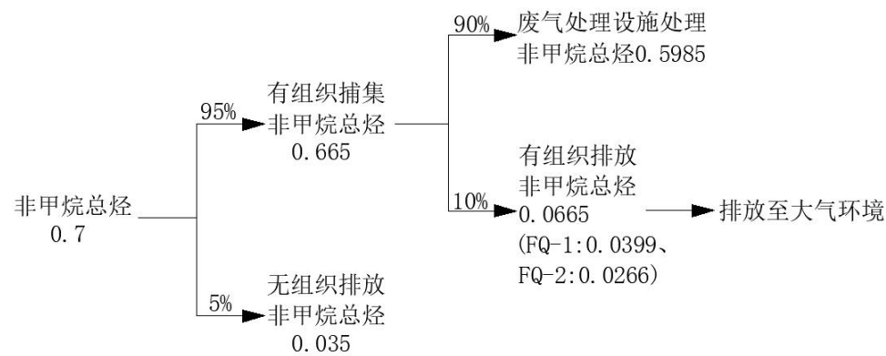
图 2-1 非甲烷总烃平衡图 (t/a)
