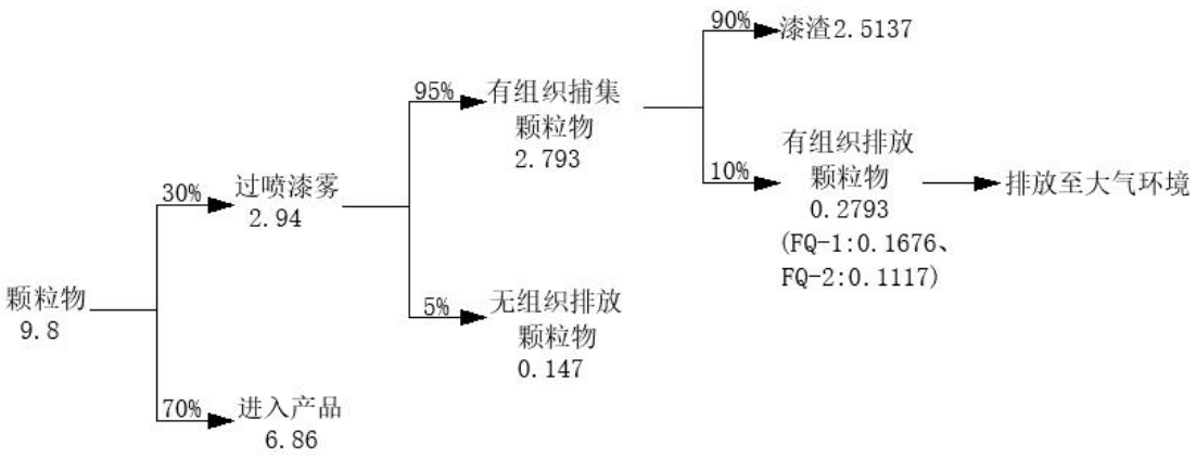
图 2-2 颗粒物平衡图 (t/a)
