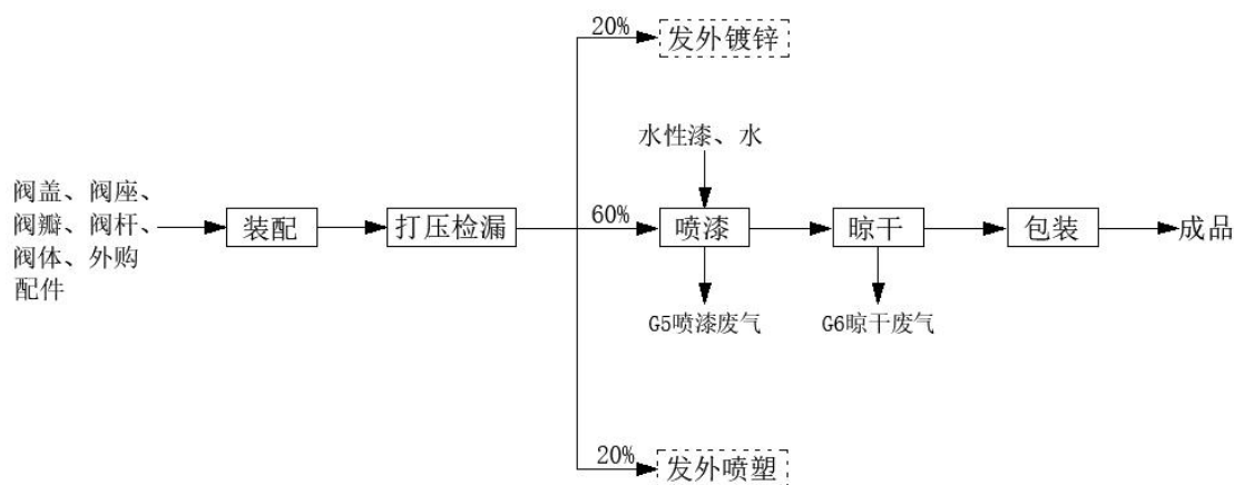
图2-9 制冷阀门生产工艺及产污流程图
