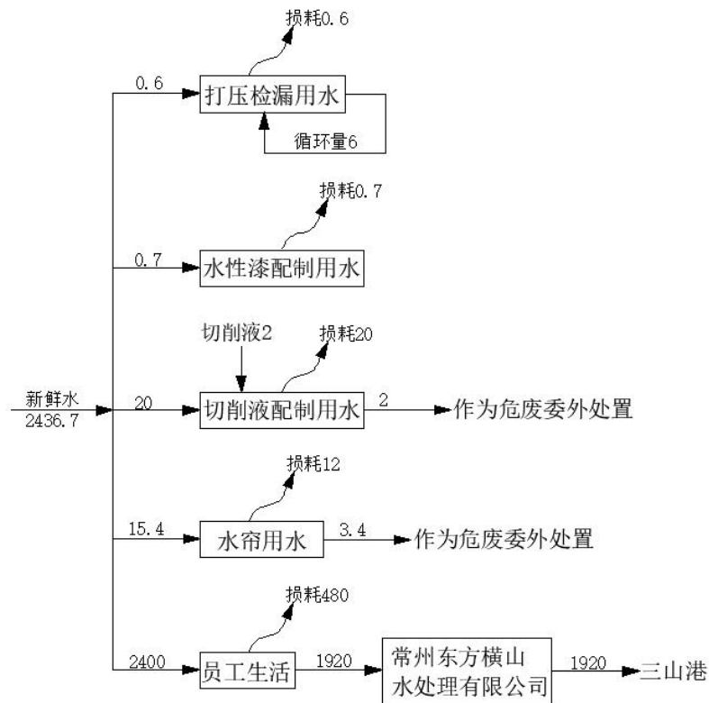
图 2-3 本项目水平衡图 (t/a)
