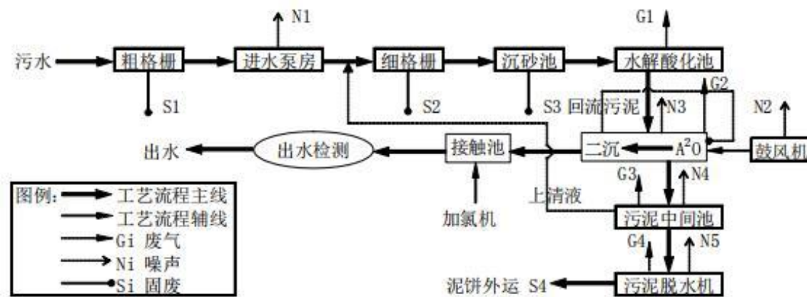
图 4-4 常州东方横山水处理有限公司污水处理工艺流程图
